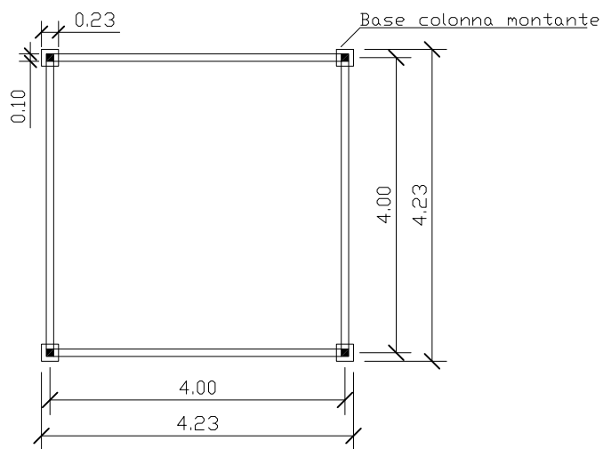
- PIANTA
