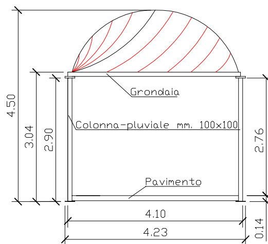
- PROSPETTO
